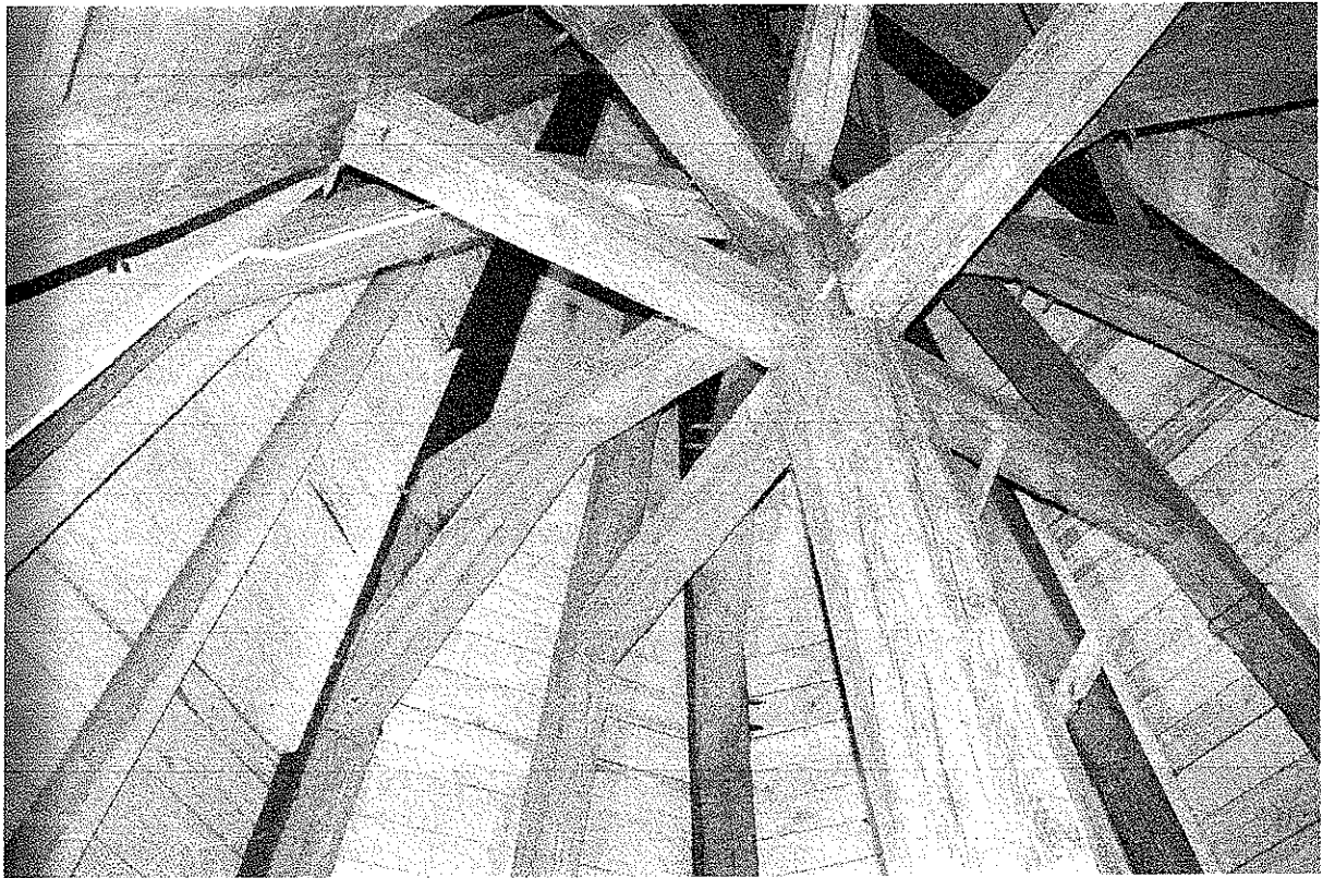
Fot. 13. Widok na konstrukcję helmu dzwonnicy
