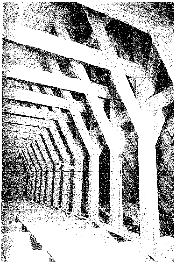
Fot. 7. Widok na wieżbę dachową i zamknięcie prezbiterium
