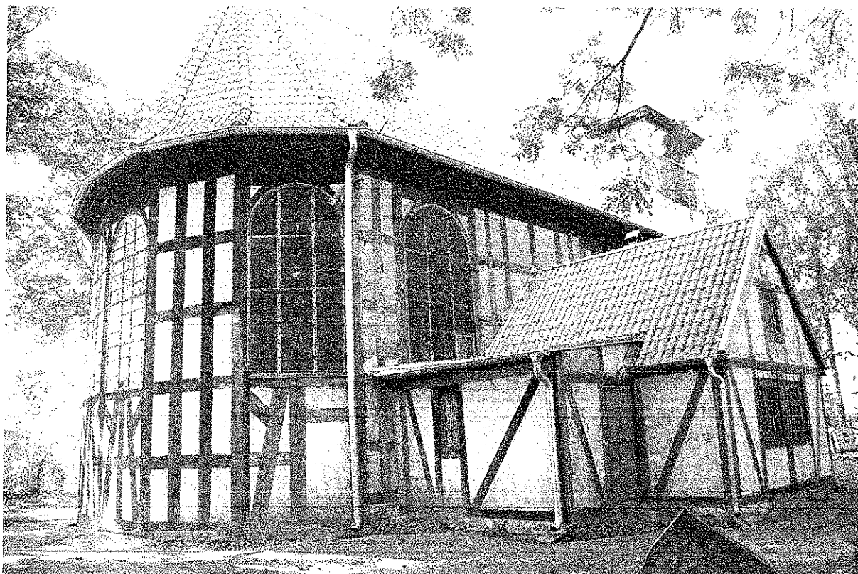
Fot. 3 . Widok na północno-wschodnią część kościoła.
