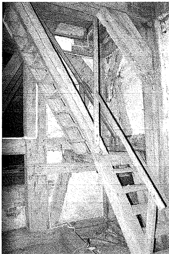
Fot. 9. Widok na konstrukcję dzwonnicy i drewniane schody
