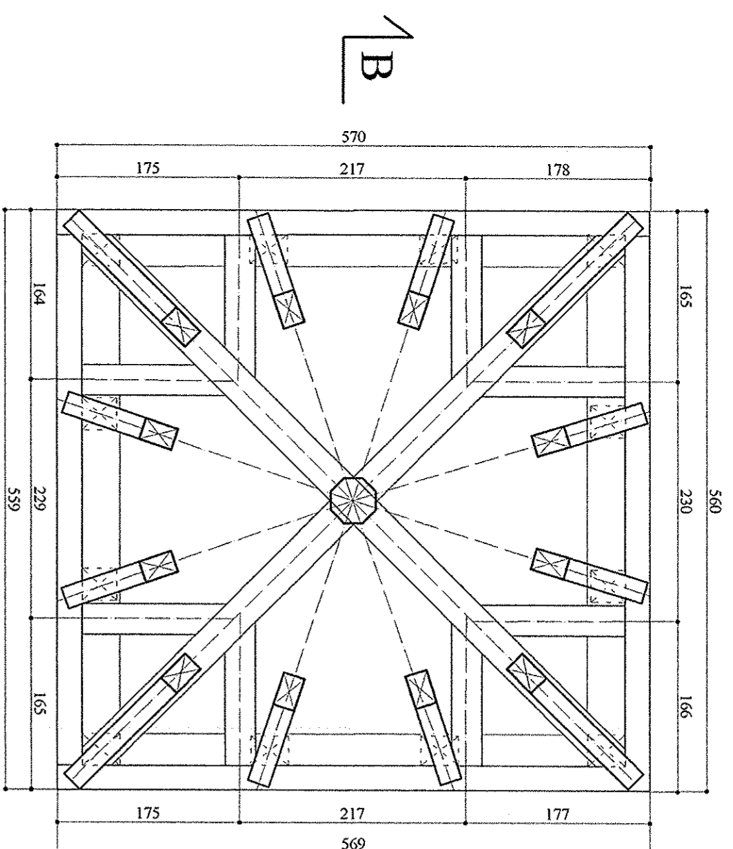
RZUT POZIOMU 4-4
