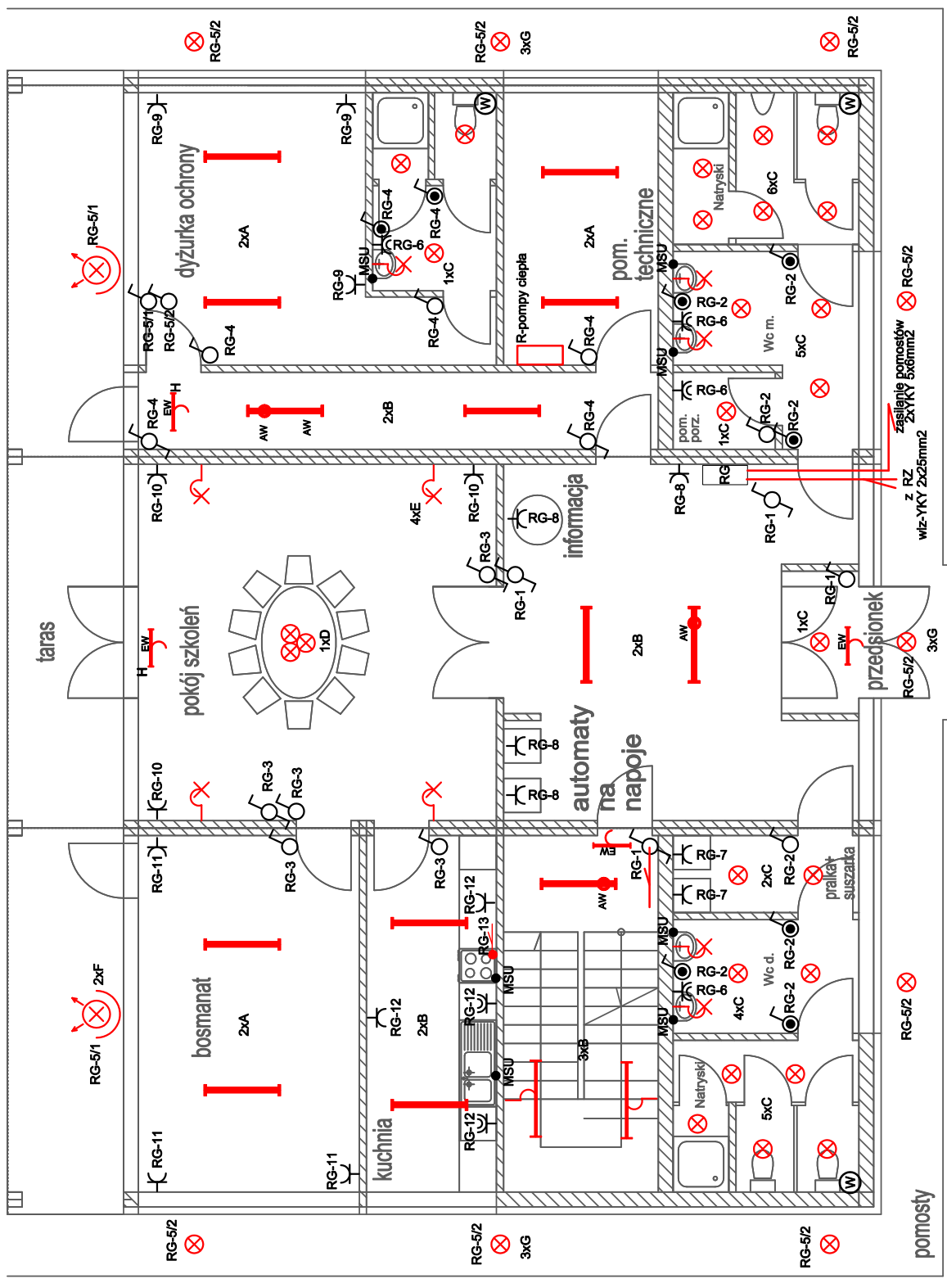
rzut parteru
