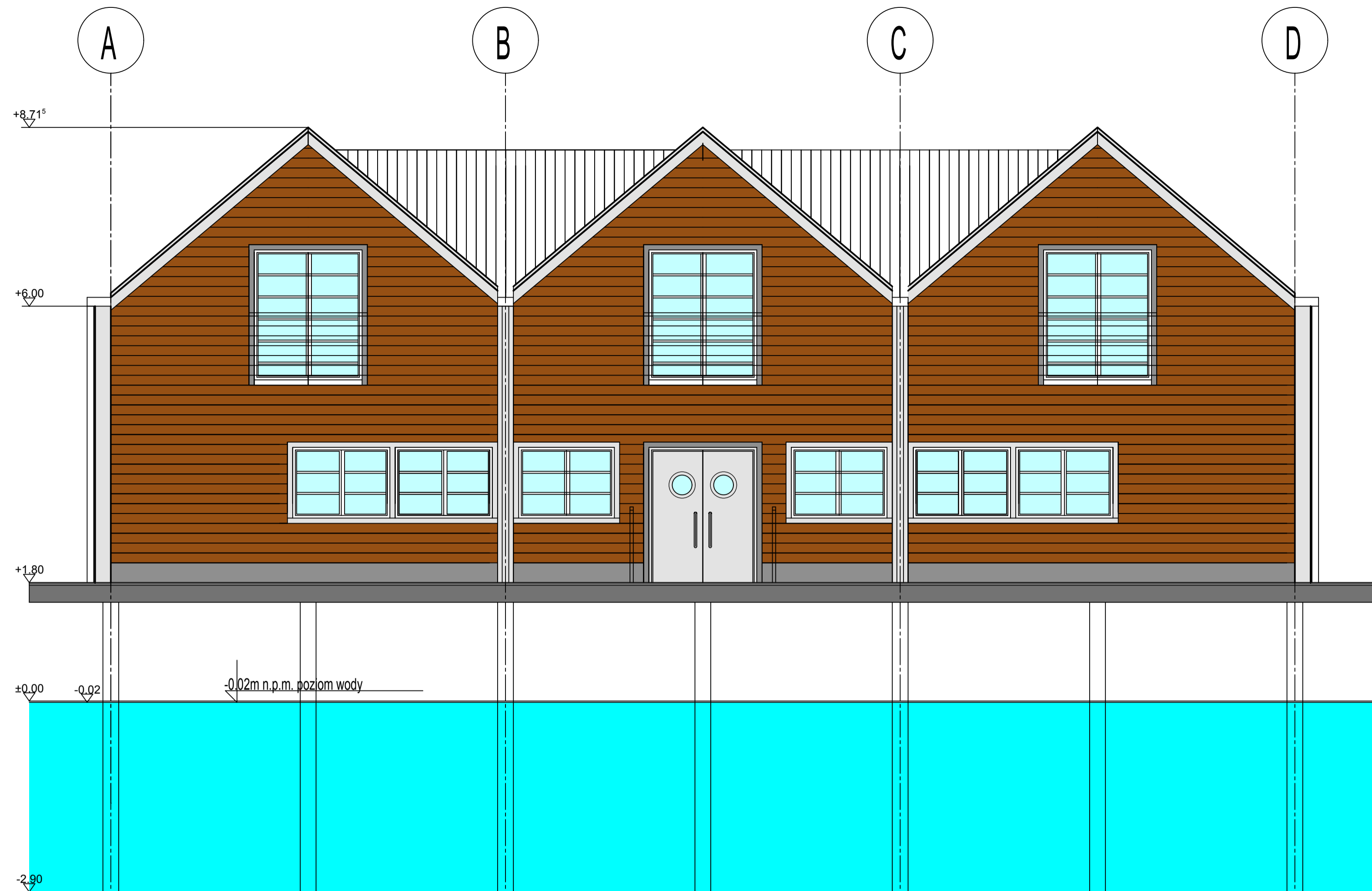
elewacja południowa
