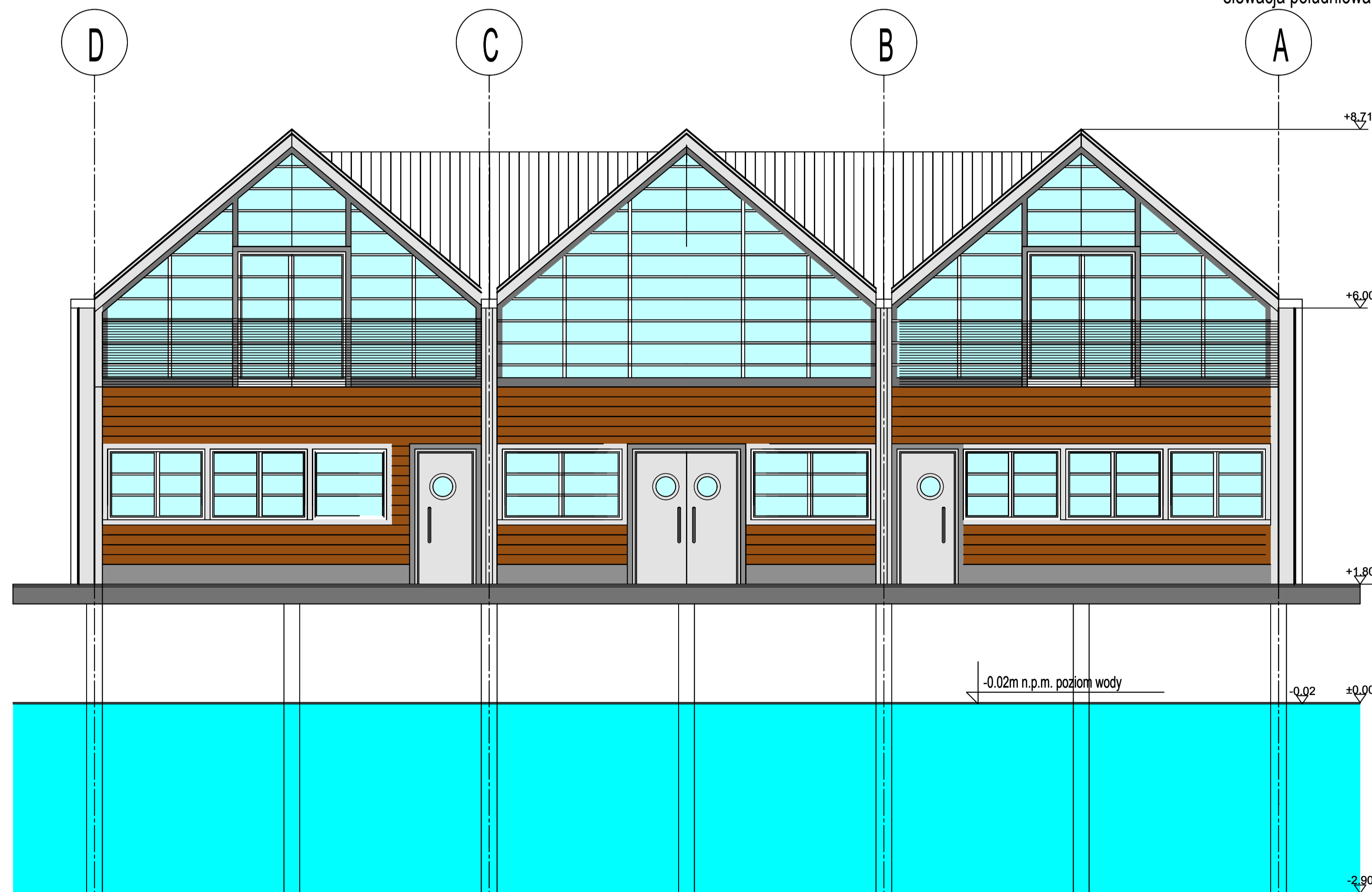
elewacja północna
