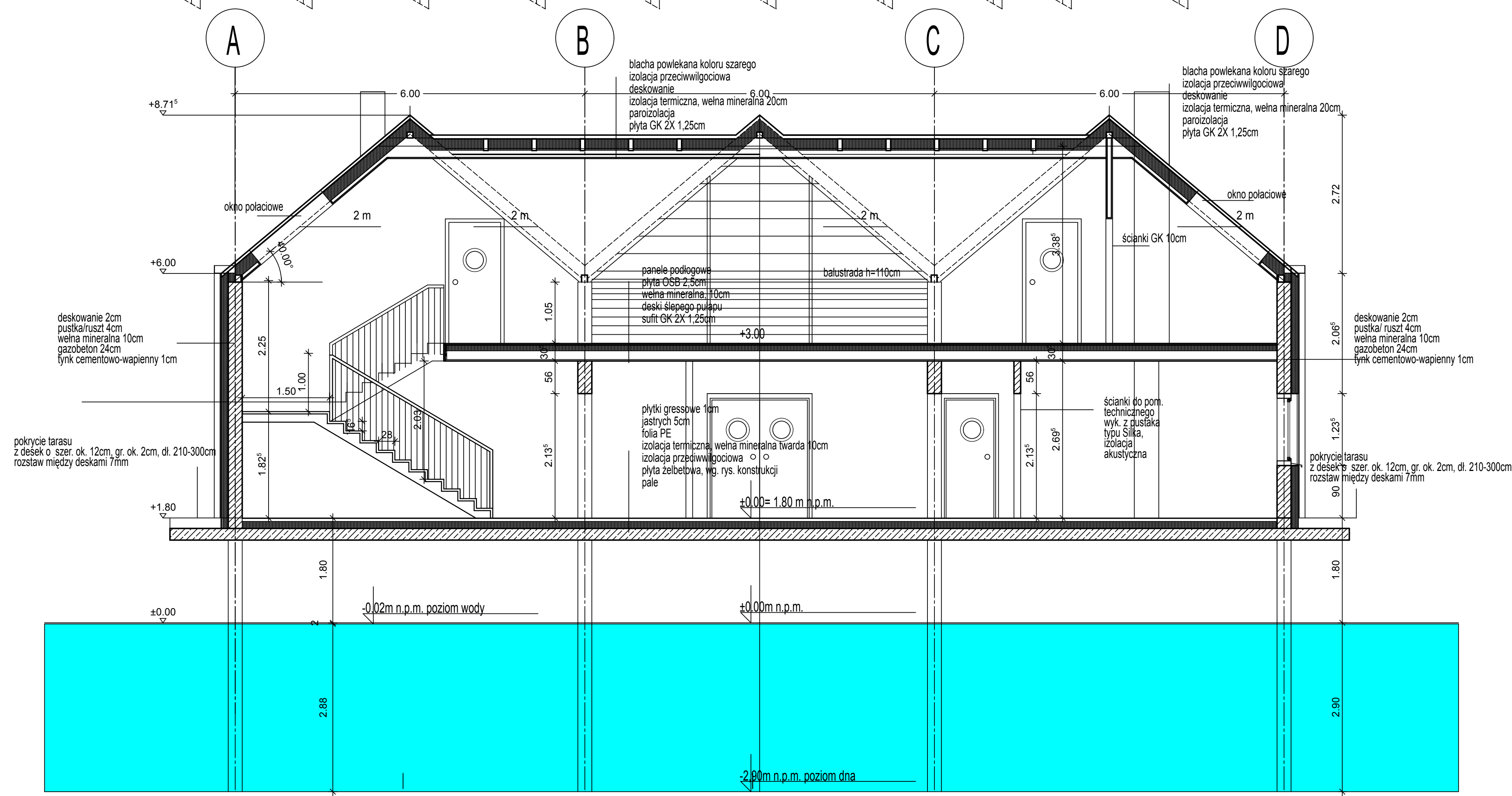
przekrój A-A
