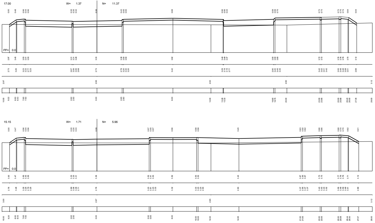
PRZEKROJE POPRZECZNE ODC. A-B-C-D ark.nr 3/8
